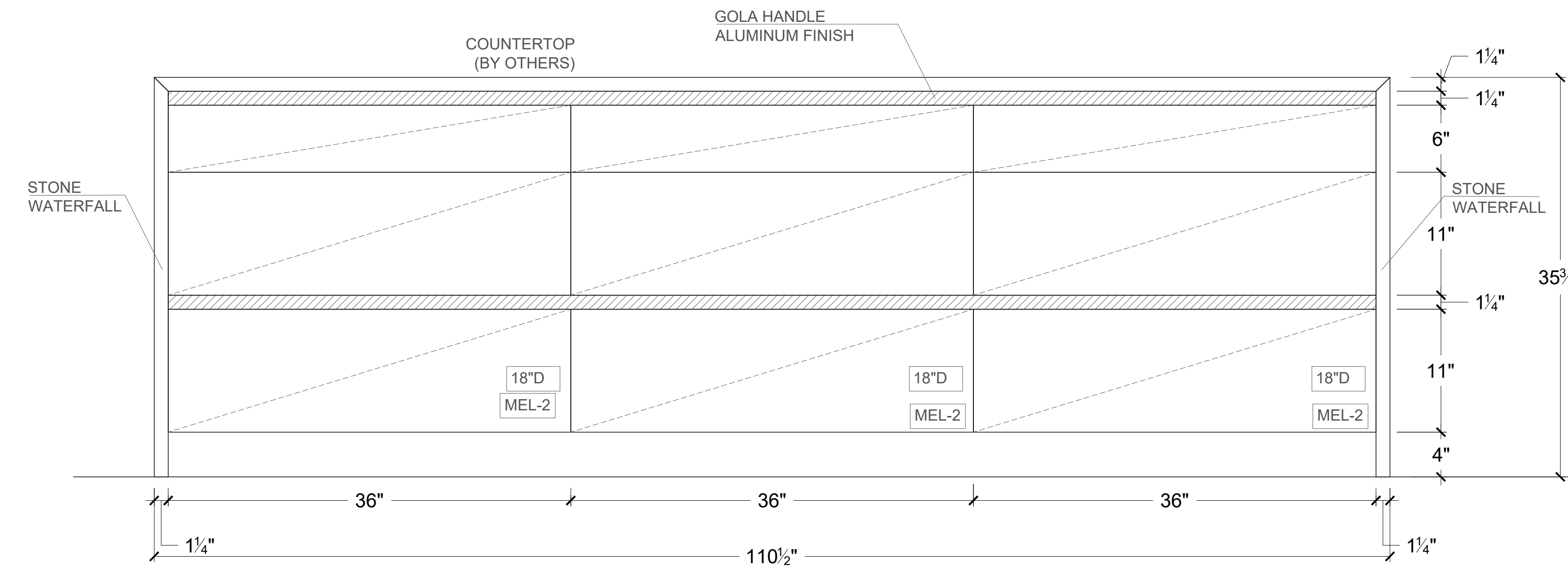
ELEVATION
