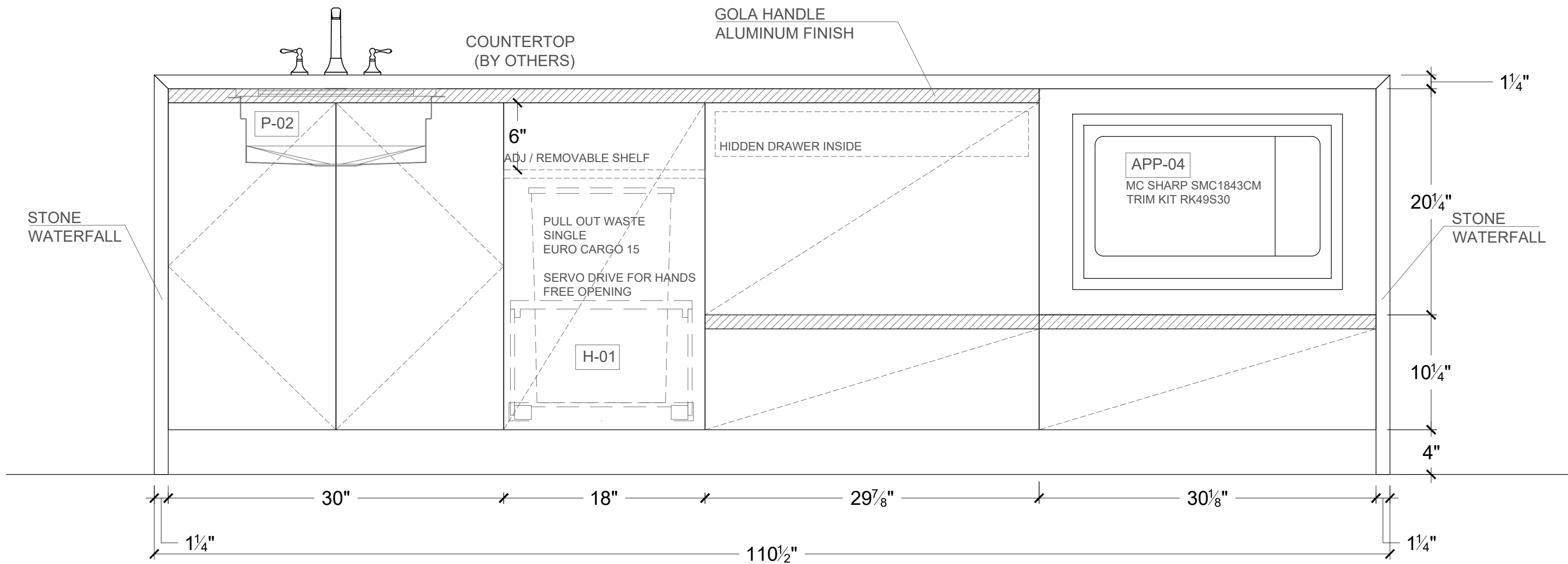
1 ELEVATION
